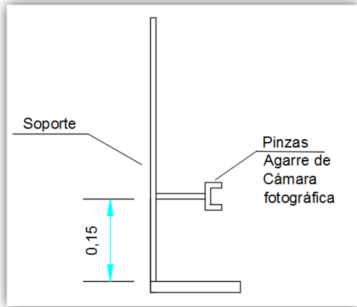
Ilustración 8. Esquema montaje fotográfico.
