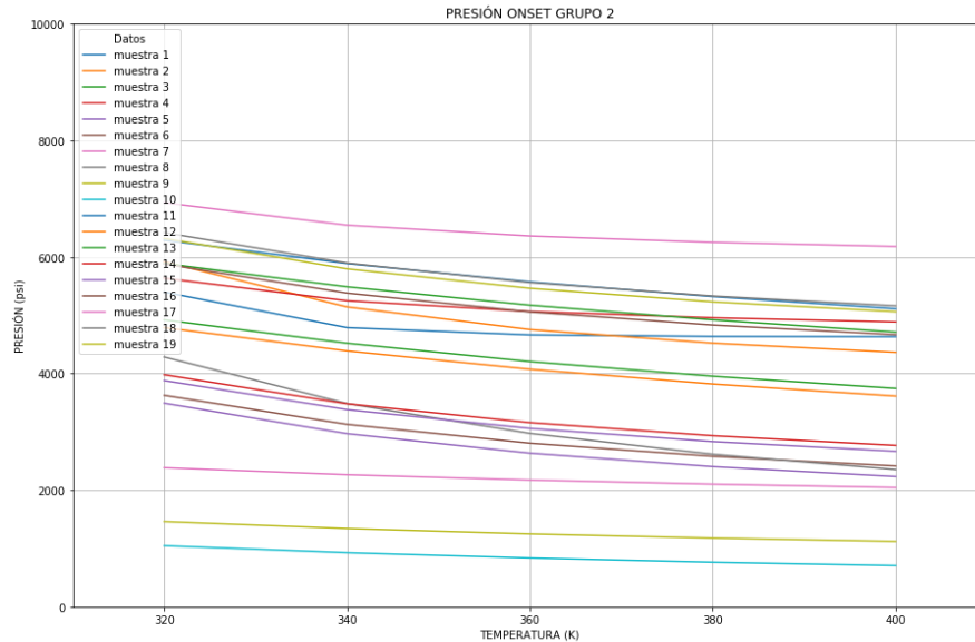
Figura 4.16 Gráfica AOP vs Temperatura Grupo 2.
