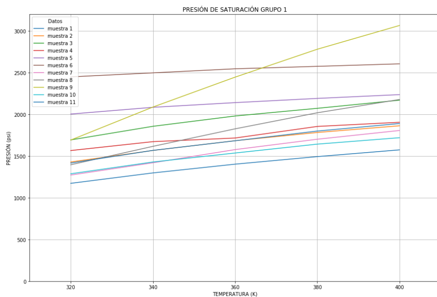
Figura 4.13 Tendencia de la presión de saturación del grupo 1 con respecto a la variación de temperatura.
