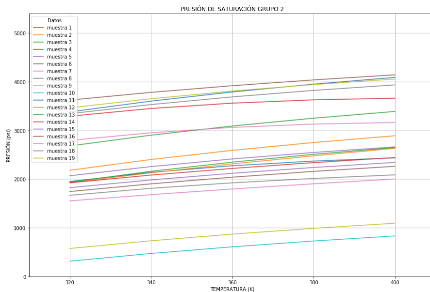
Figura 4.17 Tendencia de la presión de saturación del grupo 2 con respecto a la variación de temperatura.
