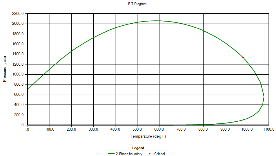
Figura 2.5 Envolvente Presión Vs Temperatura
