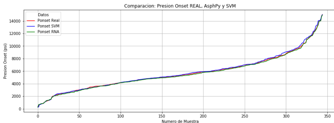
Figura 4.11 Presión real vs predicciones de los modelos de predicción.
