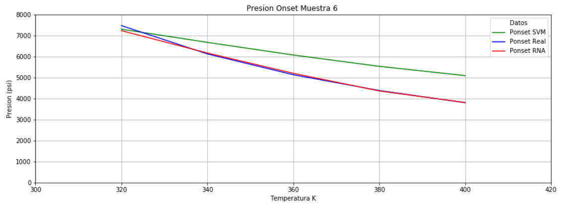
Figura 4.6 Presión vs temperatura muestra (6) presión Onset (upper).
