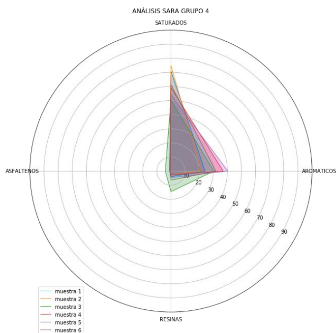
Figura 4.27 Análisis SARA del grupo 4.
