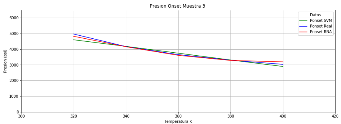
Figura 4.3 Presión vs temperatura muestra (3) presión Onset (upper).
