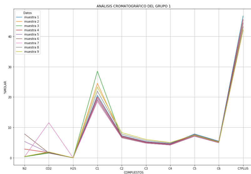
Figura 4.15 Análisis cromatográfico del grupo 1.
