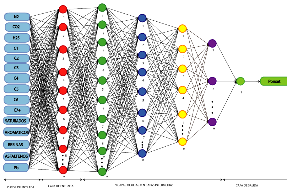
Figura 3.9 Arquitectura de la red neuronal AsphPy.
