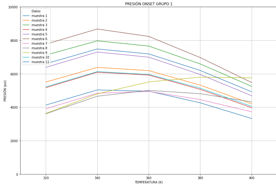
Figura 4.12 Gráfica AOP vs Temperatura Grupo 1.
