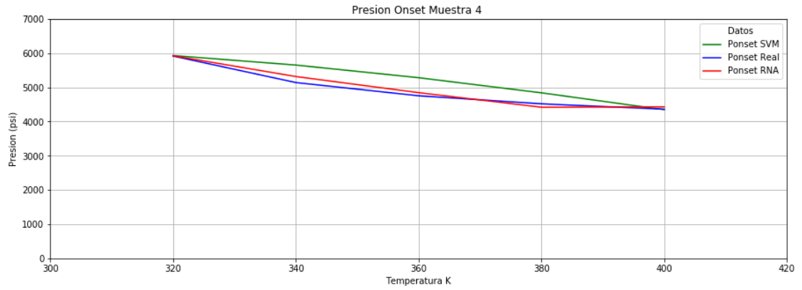
Figura 4.4 Presión vs temperatura muestra (4) presión Onset (upper).
