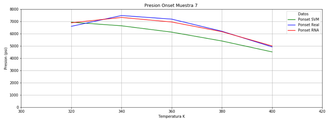
Figura 4.7 Presión vs temperatura muestra (7) presión Onset (upper).
