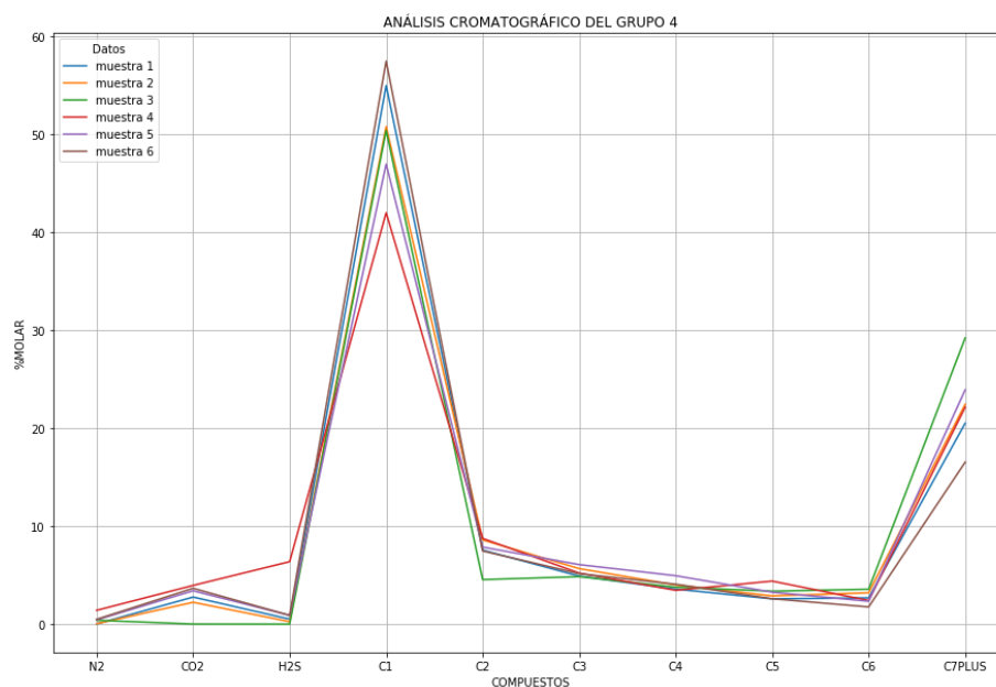
Figura 4.26 Análisis cromatográfico del grupo 4.
