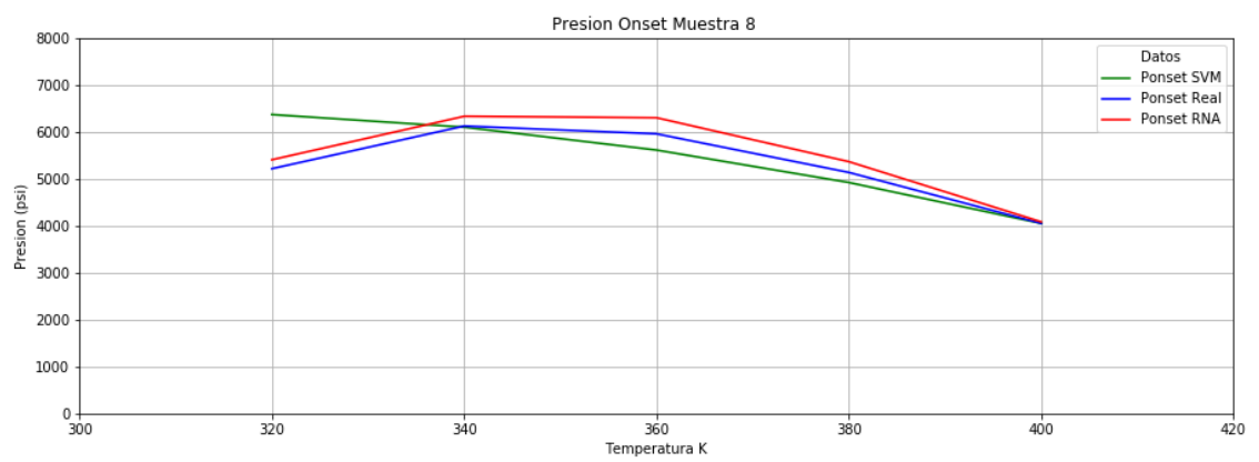
Figura 4.8 Presión vs temperatura muestra (8) presión Onset (upper).
