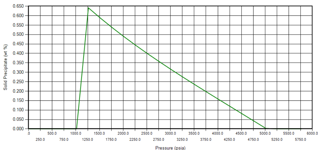
Figura 2.6 Gráfica % Asfaltenos precipitados Vs Presión.
