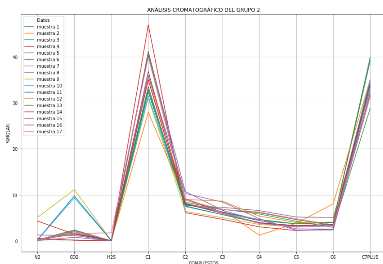
Figura 4.19 Análisis cromatográfico del grupo 2.
