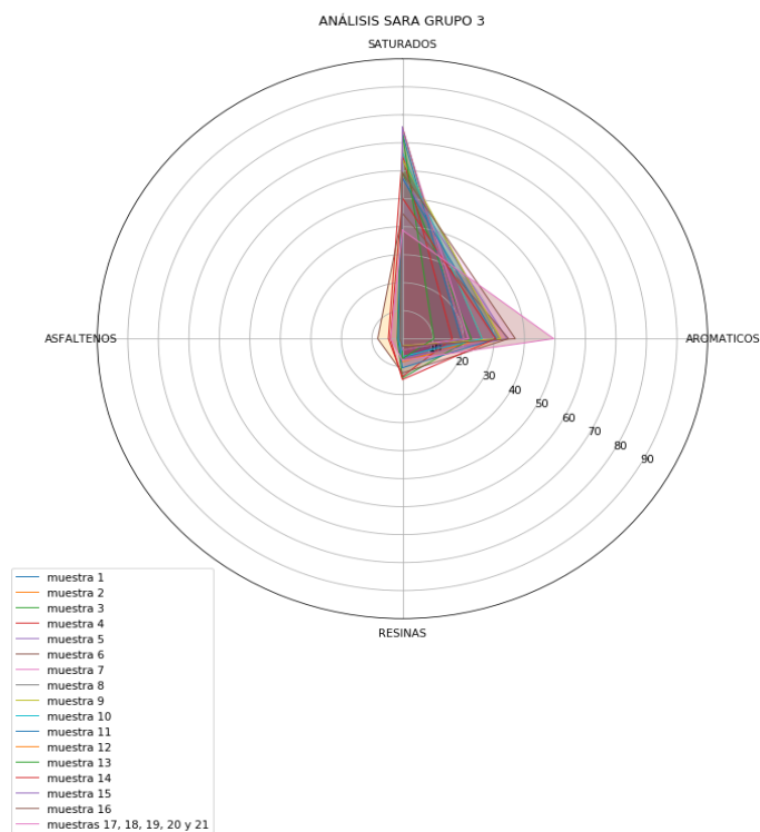
Figura 4.23 Análisis SARA del grupo 3.
