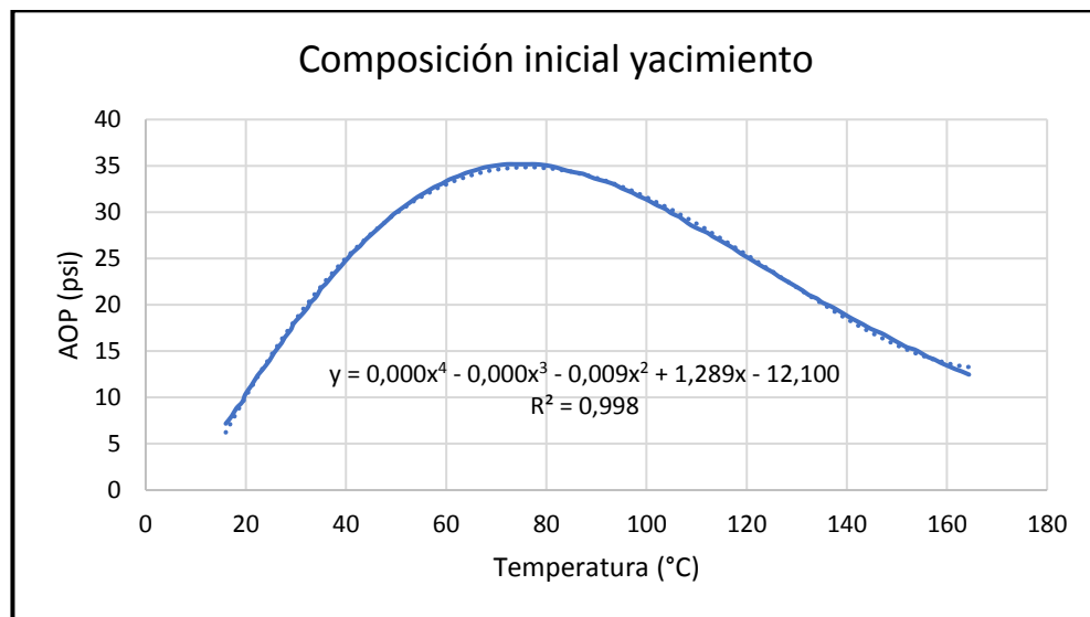
Figura 2.3 Gráfica obtenida de los puntos exportados de Digitize It.
