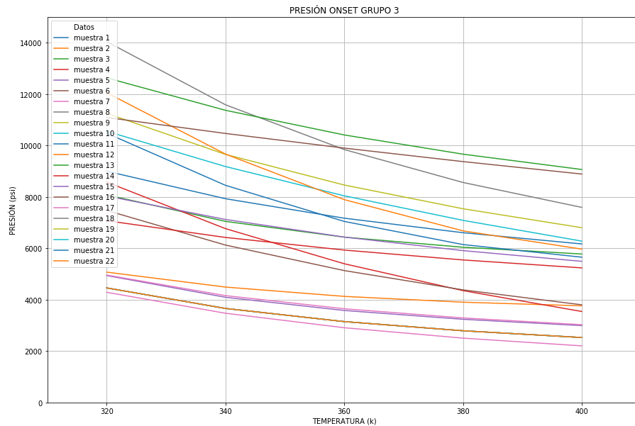
Figura 4.20 Gráfica AOP Vs Temperatura Grupo 3.
