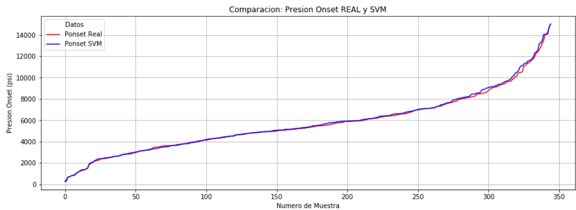
Figura 4.10 Presión real vs predicciones de las máquinas de soporte vectorial.
