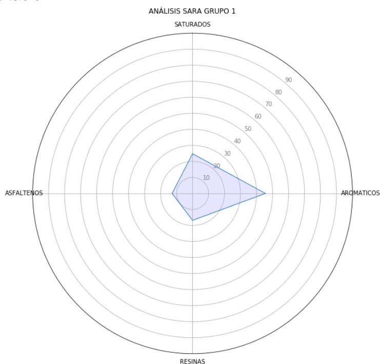
Figura 4.14 Análisis SARA del grupo 1.
