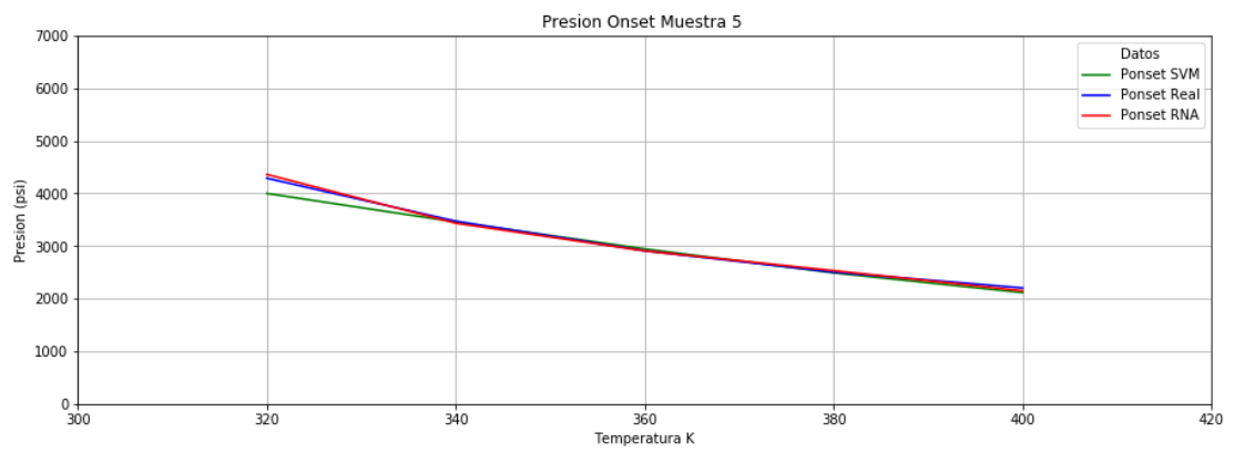
Figura 4.5 Presión vs temperatura muestra (5) presión Onset (upper).
