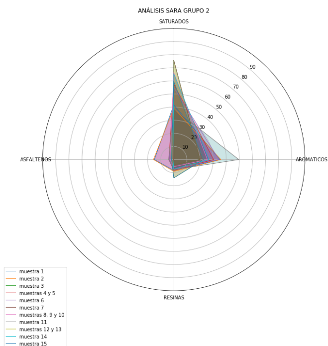
Figura 4.18 Análisis SARA del grupo 2.
