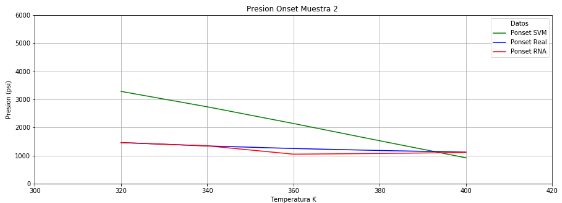
Figura 4.2 Presión vs temperatura muestra (2) presión Onset (upper).
