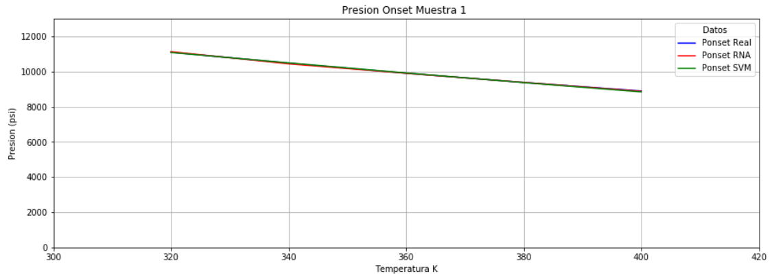
Figura 4.1 Presión vs temperatura muestra (1) presión Onset (upper).
