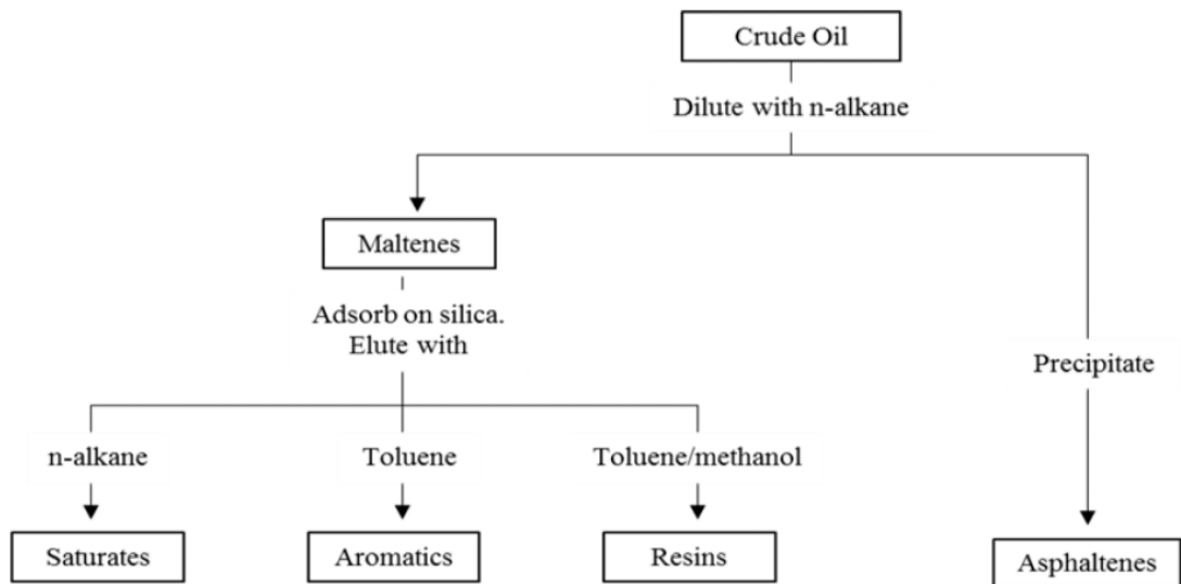
Figura 1.1. Esquema típico en separación de hidrocarburos en fracciones SARA (Al-Qasim, A., y Bubshait, A, 2017).
