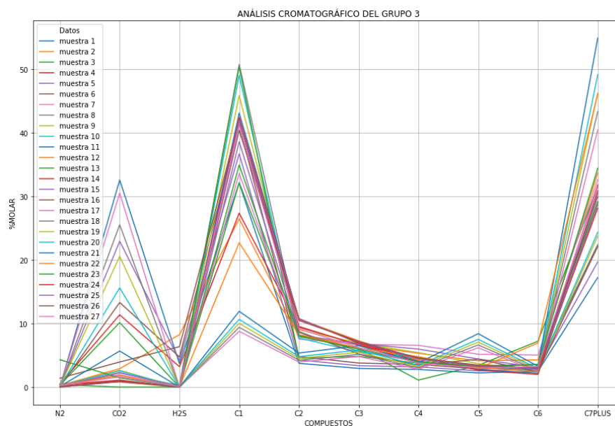
Figura 4.22 Análisis cromatográfico del grupo 3.
