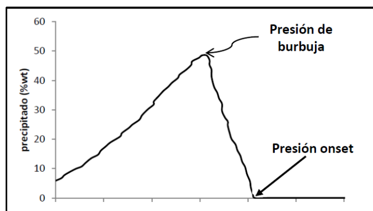
Figura 1.1 Presión Onset de precipitación de asfáltenos (Cano y Herrera, 2016)
