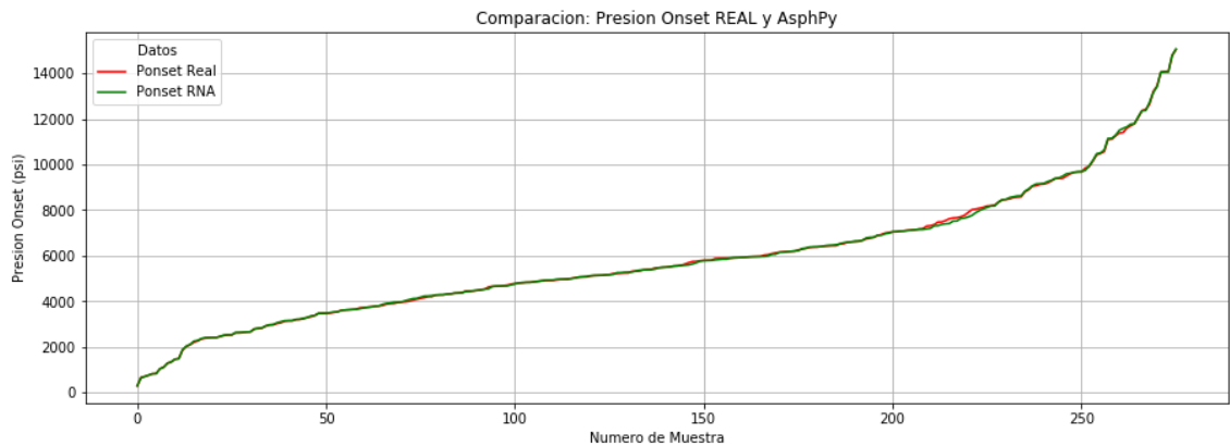
Figura 4.9 Presión real vs predicciones de la red neuronal.
