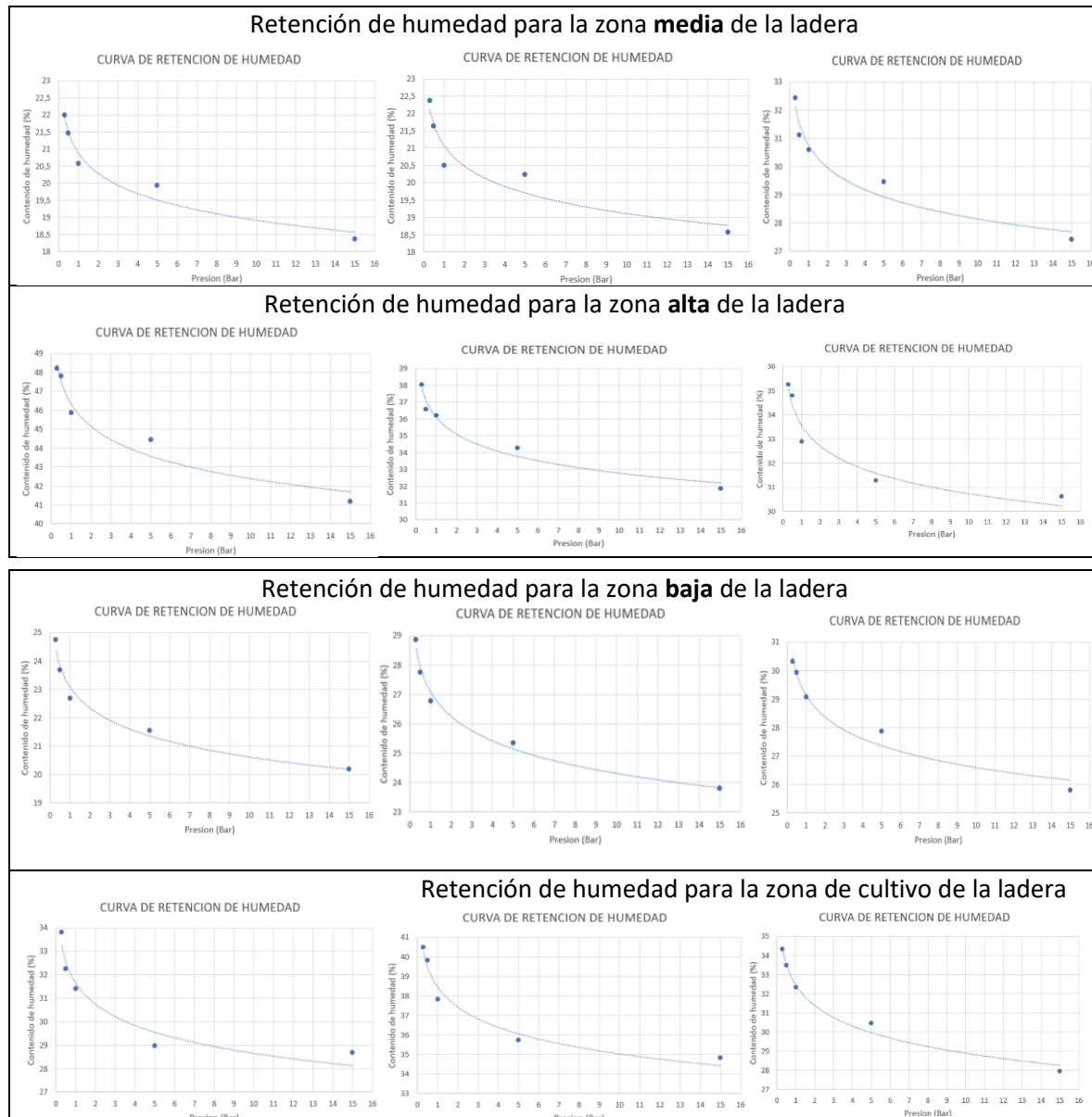
FIGURA 36. gráficas de retención de humedad para cada zona de ladera.
