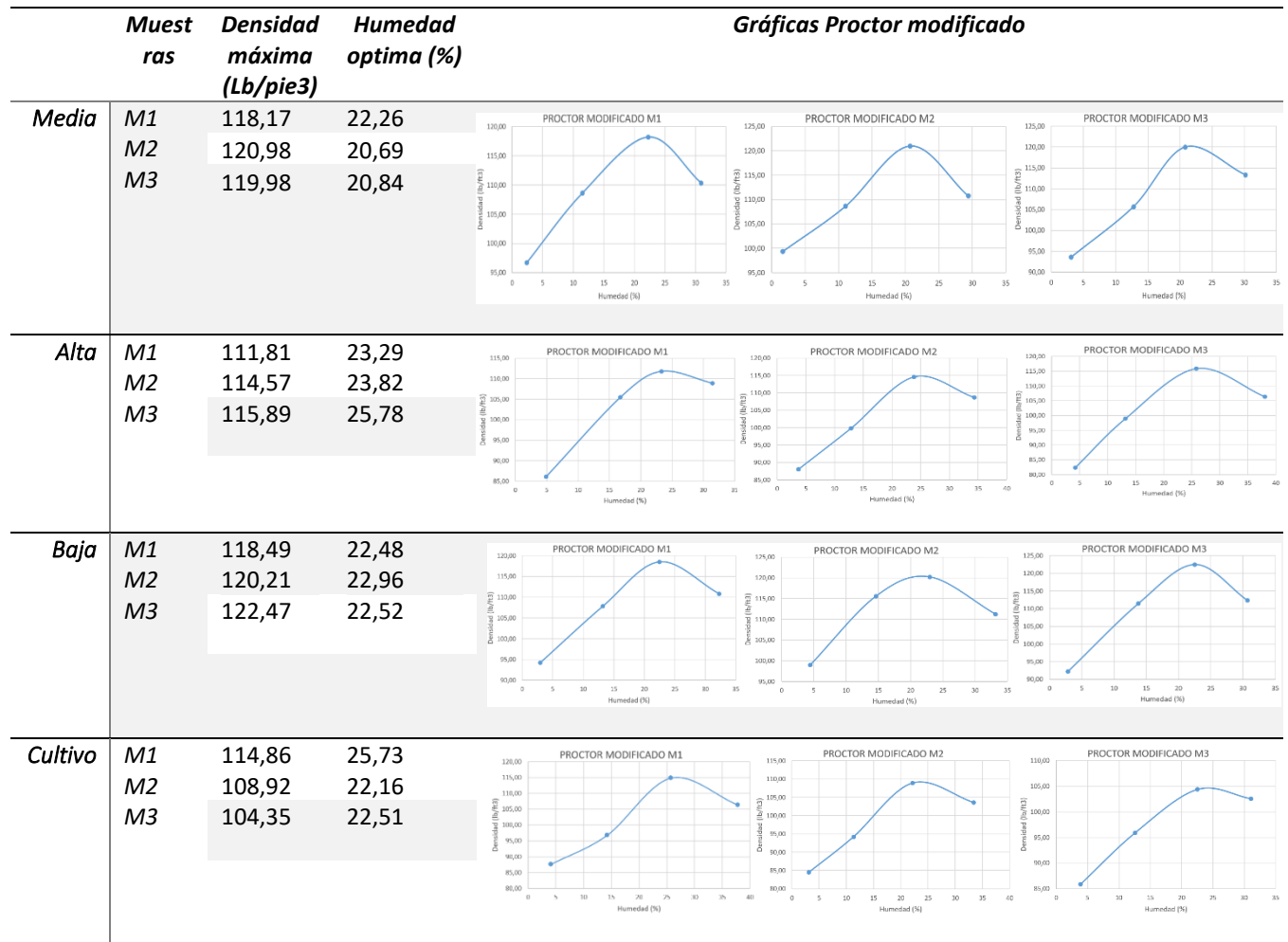
FIGURA 34. gráficas de proctor modificado para cada zona de ladera.
