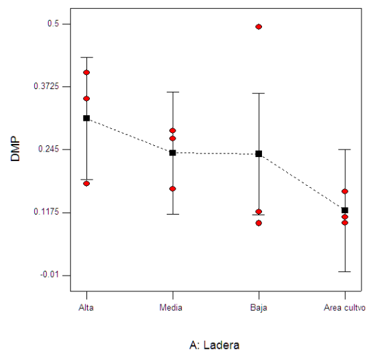
FIGURA 29. Diámetro medio ponderado en las diferentes zonas de ladera.
