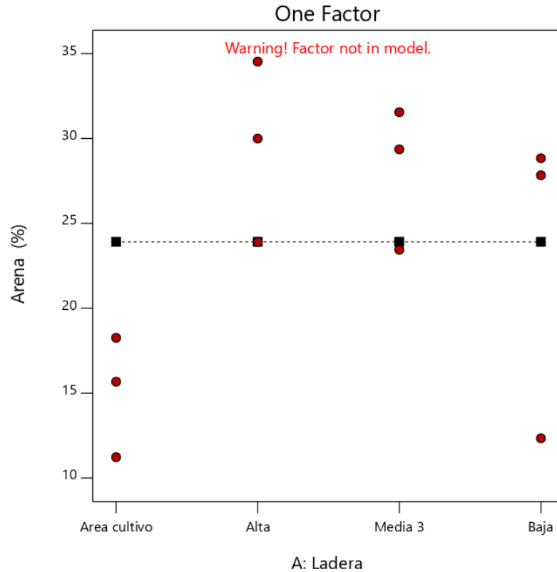
FIGURA 30. Porcentaje de arena pérdida en las diferentes zonas de la ladera.
