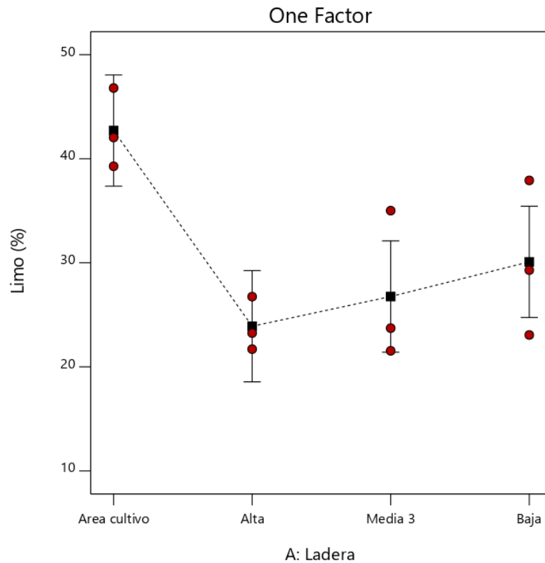
FIGURA 32. Porcentaje de limo perdido en las diferentes zonas de la ladera.
