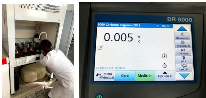
FIGURA 13. Procedimiento para la determinación del carbono orgánico. Fuente: autores.
